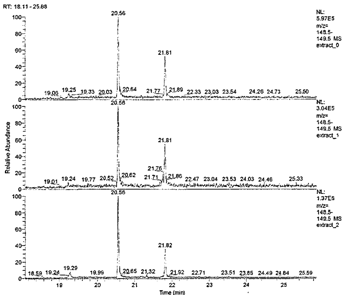
Рис. 2. Масс-хроматограммы образцов холостого эксперимента и образцов экстрактов фталатов из ПТЭ-бутылок образцов №1 и 2 (сверху вниз) по иону 149 (характерному для фталатов). Пики 20,5 и 21,8 соответствуют динозбутилфталату и дибутилфталату соответственно.
